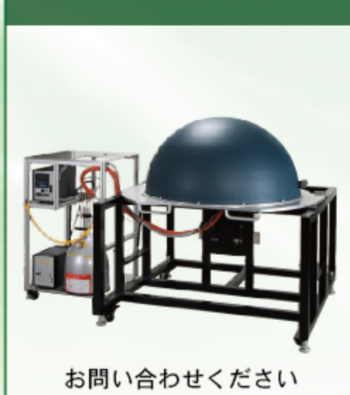
全光束測定システム
